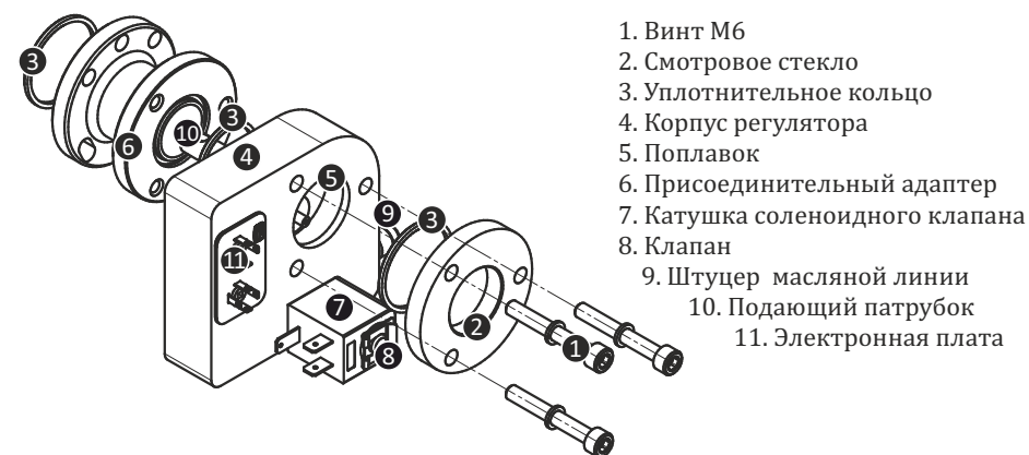
Рис.2. Монтажный чертеж
